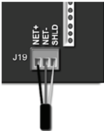
Fig. 16 - Network Wiring
